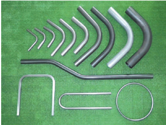
様々な種類・サイズのパイプ曲げ加工が可能
